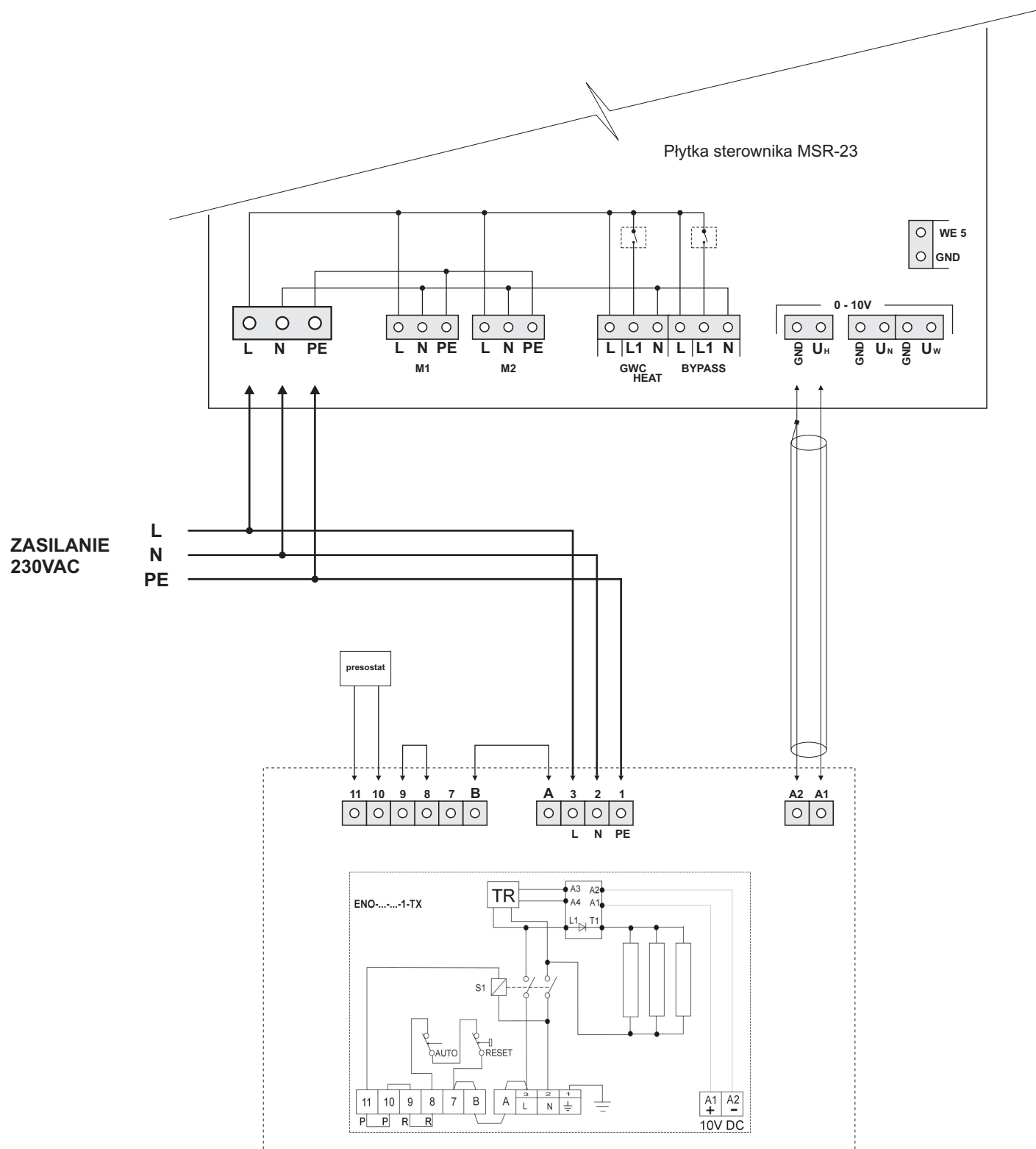
Elektryczna nagrzewnica wtórna z pulserem typu ENO-.....-X
